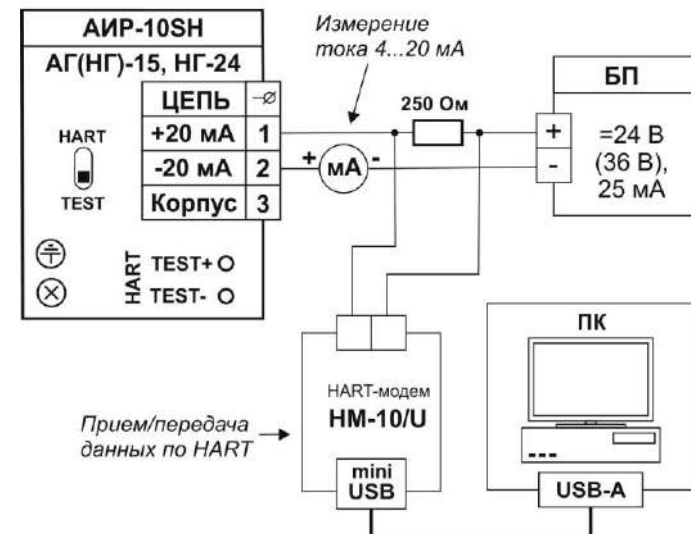
Рисунок А.17 HART-модем. 2 вариант
